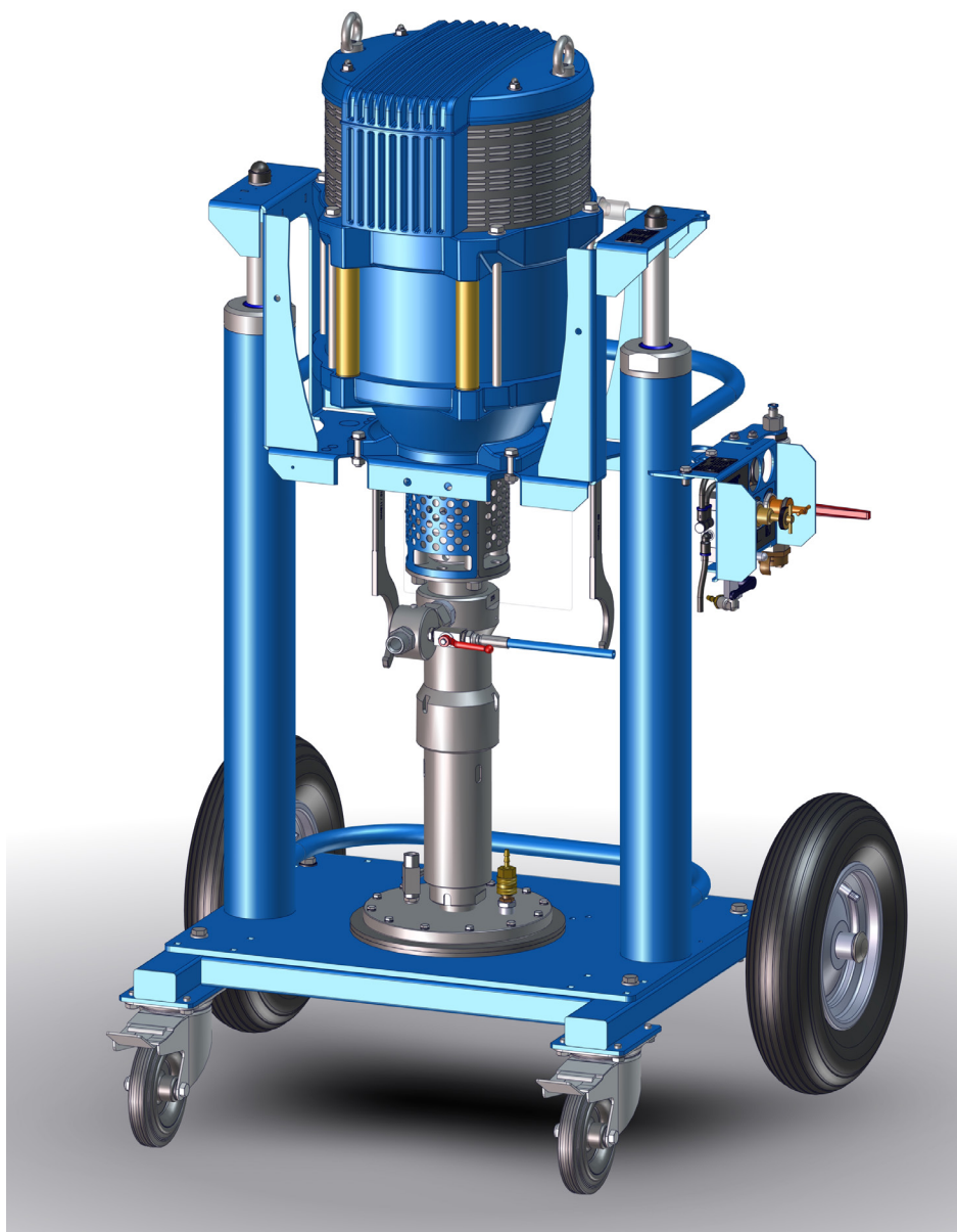
WIWA Airless 333075 R/ZSR für GRIWECOLOR
